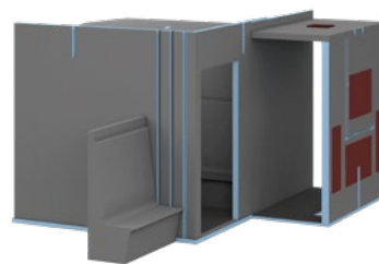
Hamam, banquette et douche modulaire Construction d'un espace bien-être privé avec hammam, douche sensorielle à jets et pédiluve
