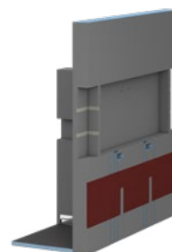
Module en T à trois côtés Solution système pour toilettes, douche et lavabo avec composants techniques et renforts
